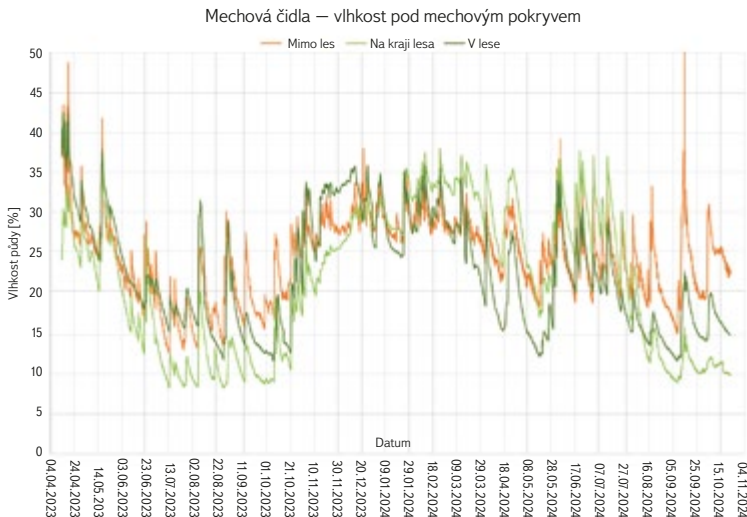
Obr. 3. Dynamika objemové půdní vlhkosti pod mechovým pokryvem v lese, na okraji lesa a mimo les Fig. 3. Volumetric soil moisture under moss cover in the forest, forest edge, and outside the forest
