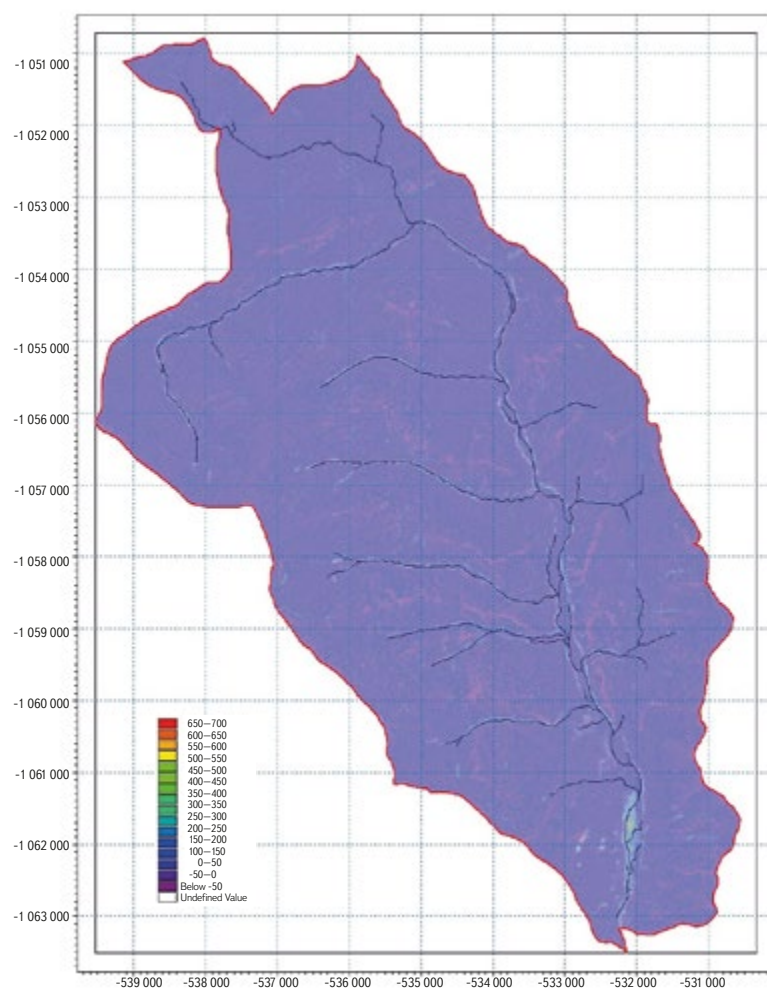
Obr. 6. Hodnoty return flow (exfiltrace) pro epizodu 14.–16. září 2024 simulované modelem MIKE SHE
