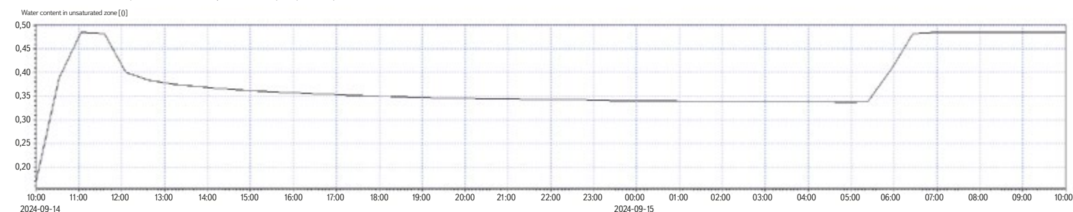
Obr. 4. Simulace dynamiky povrchové (hloubka 10 cm) objemové půdní vlhkosti v modelu MIKE SHE pro epizodu 14.–16. září 2024
