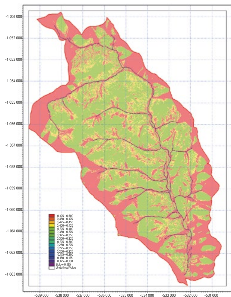
Obr. 5. Hodnoty objemové půdní vlhkosti pro epizodu 14.–16. září 2024 simulované modelem MIKE SHE
