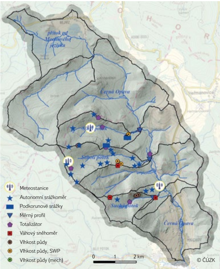
Obr. 1. Rozmístění čidel a vodoměrných profilů na pilotních povodích Suchého, Sokolího a Slučího potoka Fig. 1. Distribution of sensors and water gauges on the pilot catchments of Suchý, Sokolí, and Slučí brooks
