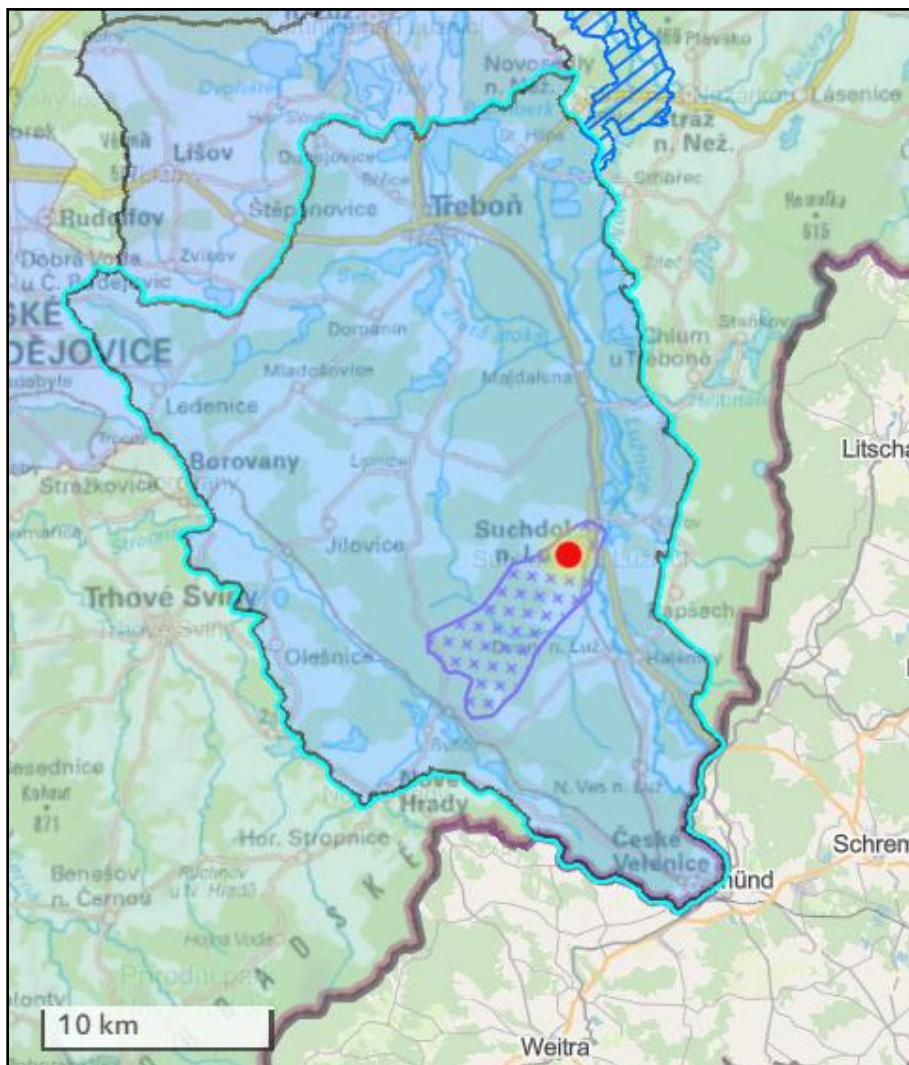
Obr. 4. Vymezení povodí odběru (fialově označené území) ČEVAK Suchdol n/Lužnicí (ID Surová voda : 11300600) na základě podkladů hydraulického modelu firmy Progeo, s. r. o., a jeho zařazení do širšího kontextu příslušného hydrogeologického rajonu Třeboňská pánev – jižní část (modře vysvícené území)
