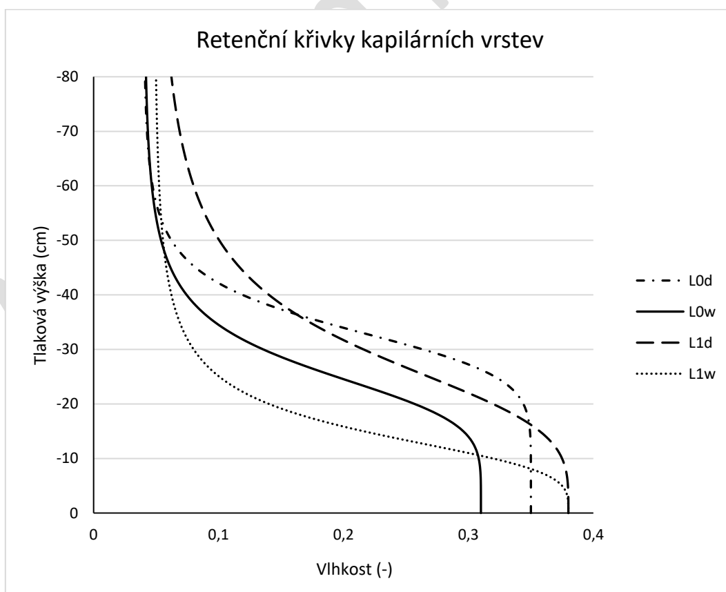
Obr. 2. Hlavní drenážní a hlavní zvlhčovací větve retenčních křivek reálného (L 0 ) a vygenerovaného (L 1 ) materiálu kapilární vrstvy
