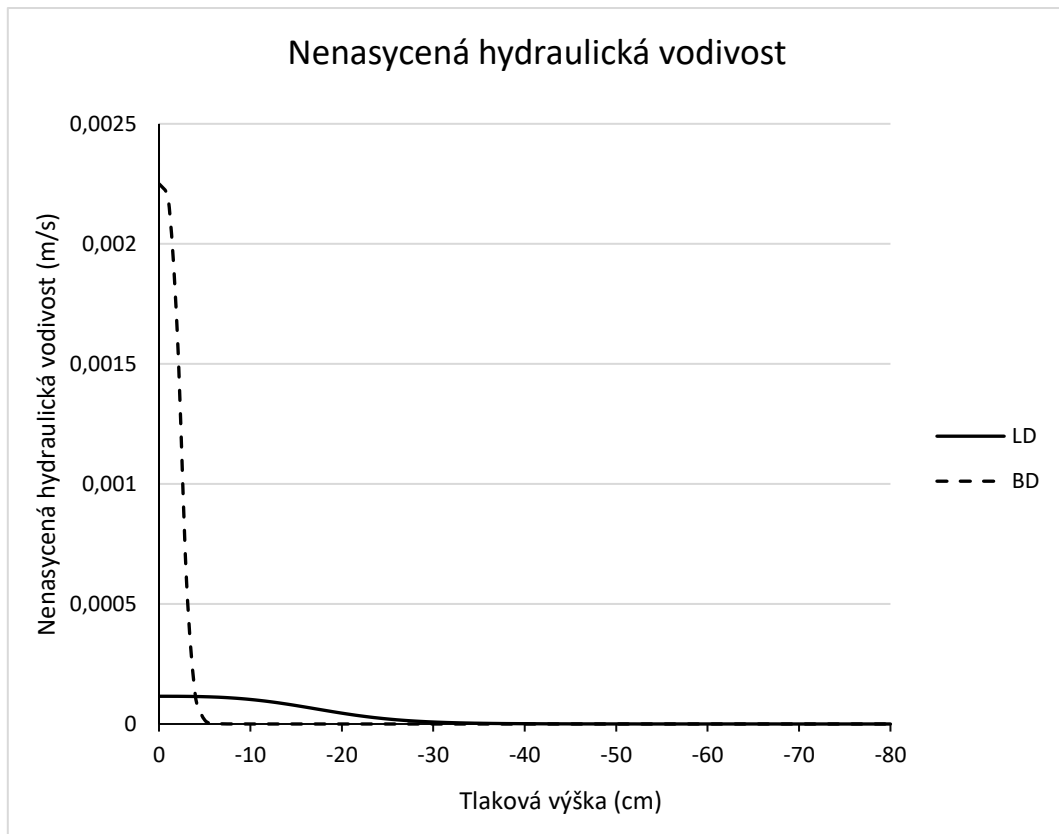
Obr. 1. Nenasycená hydraulická vodivost kapilární bariéry. Křivky závislosti nenasycené hydraulické vodivosti na tlakové výšce pro kapilární vrstvu LD a kapilární blok BD. Data odpovídají drenážní větvi retenční křivky
