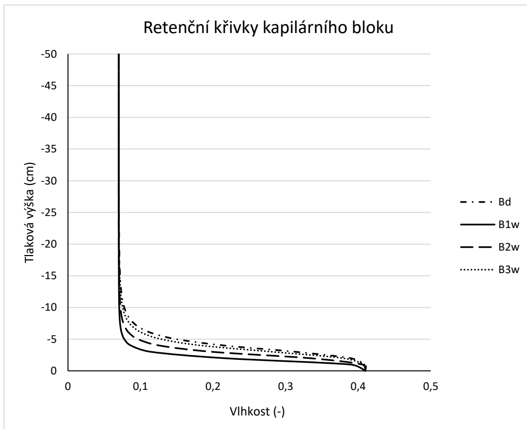
Obr. 4. Retenční křivky kapilárního bloku s odlišnými hodnotami parametru \alpha^w . Porovnání retenční křivky kapilárního bloku pro drenážní větev BD a tří variant B1w, B2w a B3w pro zvlhčovací větev reflektující změnu parametrem \alpha_w
