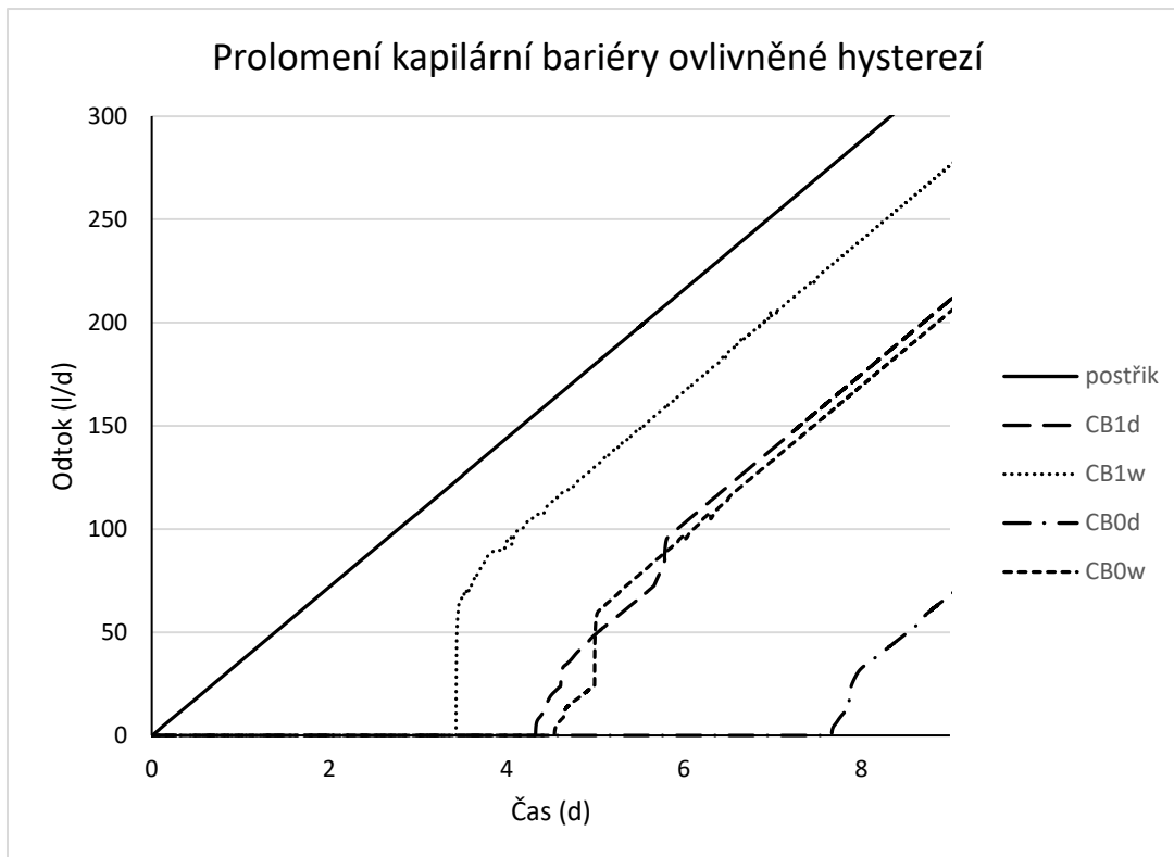
Obr. 6. Účinnost kapilární bariéry ovlivněná hysterezí. Graf znázorňuje lineárně narůstající postřik stejný pro všechny simulace, odtok z kapilárního bloku CB0d a CB0w pro drenážní a zvlhčovací větev retenční křivky výchozí kapilární bariéry a CB1d a CB1w pro drenážní a zvlhčovací větev retenční křivky varianty 1 hypotetické kapilární bariéry podle Scotta et al. [14]
