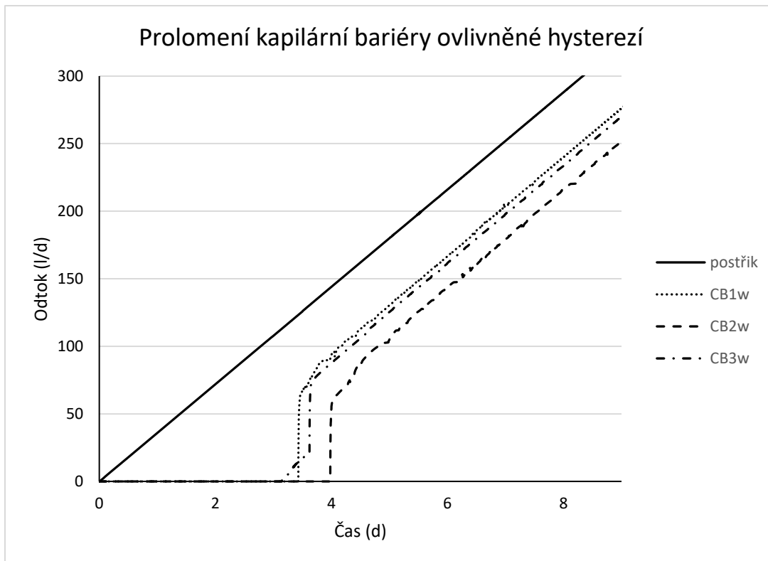
Obr. 7. Účinnost kapilární bariéry v závislosti na volbě parametru \alpha^w zvlhčovací větve retenční křivky. Postřik v grafu znázorňuje lineárně narůstající intenzitu postřiku, zvlhčovací křivky 1, 2 a 3 odpovídají odtoku z kapilárního bloku pro tři varianty výpočtu \alpha^w zvlhčovací větve retenční křivky
