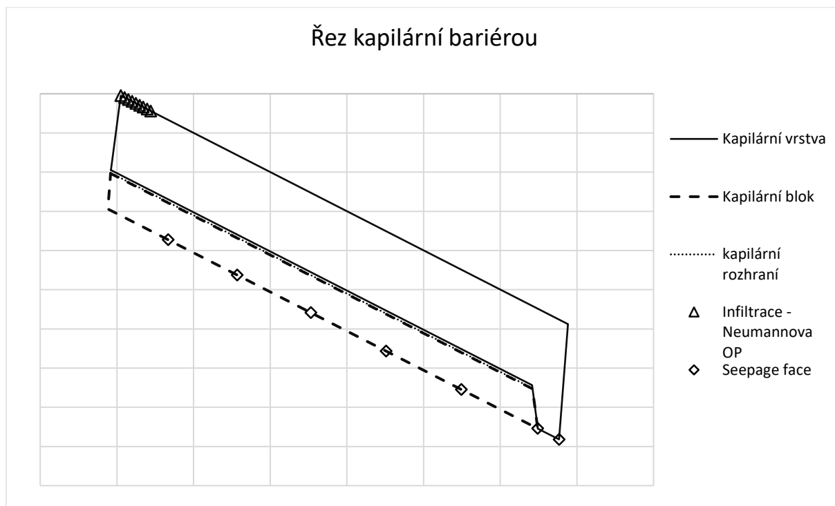
Obr. 5. Řez kapilární bariérou s vyznačenými okrajovými podmínkami pro infiltraci odpovídající nenulové Neumannově okrajové podmínce a okrajová podmínka drenáže z kapilárního bloku Seepage face. Na zbývajícím části hranice je nulová Neumannova okrajová podmínka. Délka kapilární bariéry je 6 m a výška 6 cm
