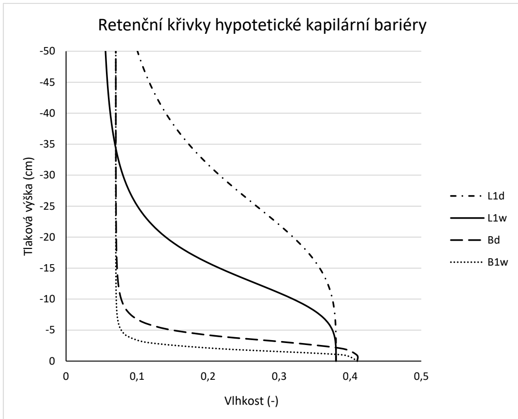
Obr. 3. Hystereze retenčních křivek kapilární vrstvy a kapilárního bloku hypotetické kapilární bariéry. Křivky L1d a Bd znázorňují drenážní větev retenčních křivek kapilární vrstvy a kapilárního bloku, L1w a B1w zobrazují zvlhčovací větev retenční křivky kapilární vrstvy a kapilárního bloku
