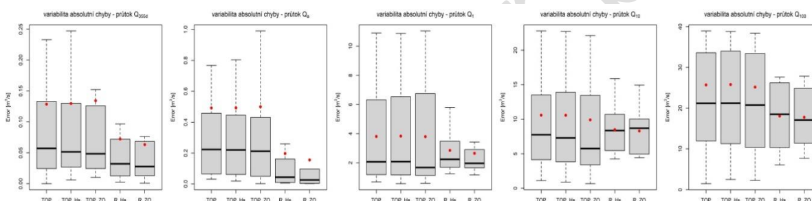
Obr. 4. Grafické znázornění variability chyb dosažených porovnáváním metodami pro jednotlivé hodnocené průtoky
