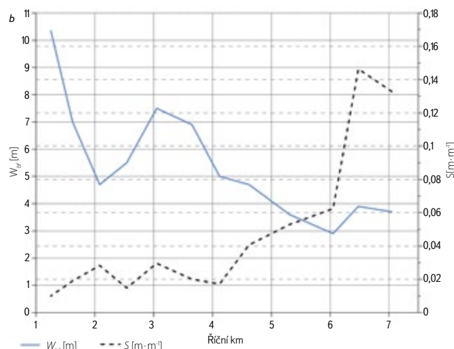
Obr. 3. a) Poproudový vývoj zrnitosti sedimentů D_{25} , D_{50} , D_{95} a SPI; b) poproudový vývoj šířek ( W_{cr} ) a sklonů ( S ) hlavního koryta Slavíče Fig. 3. a) Downstream grain size trends of sediments D_{25} , D_{50} , D_{95} and SPI; b) downstream trends of width ( W_{cr} ) and slope ( S ) of the Slavice channel
